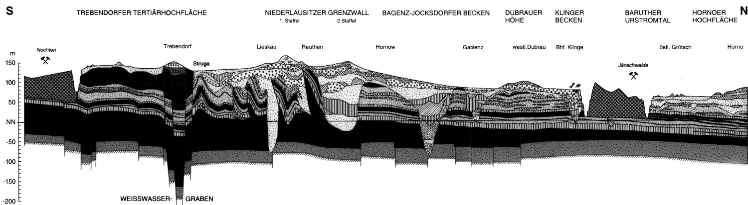
Regionalgeologischer Schnitt durch das Tertiär und Quartär (Känozoikum) des Niederlausitzer Braunkohlenreviers, 25fach überhöht (W. Nowel 1992)
